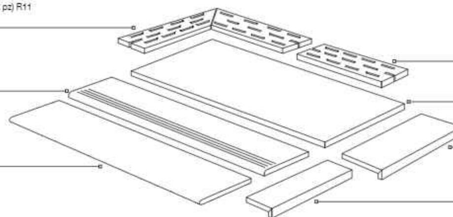
Griglia per Piscina R11 20x60 . 8"x24" RETT
